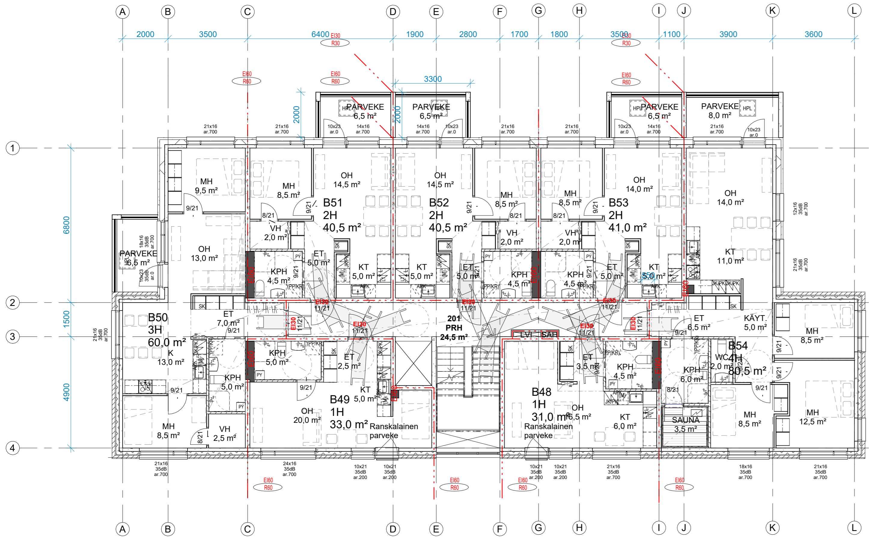
KERROKSET 2-4 1 : 100
